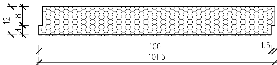
Przekrój
