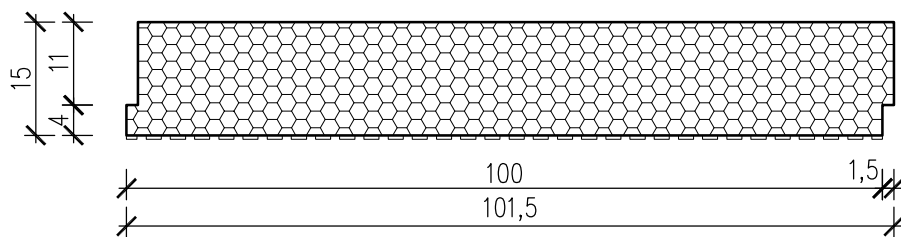
Przekrój
